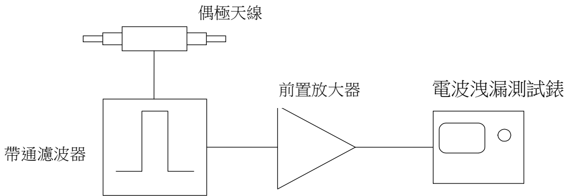
圖 1 電波洩漏測試裝置
