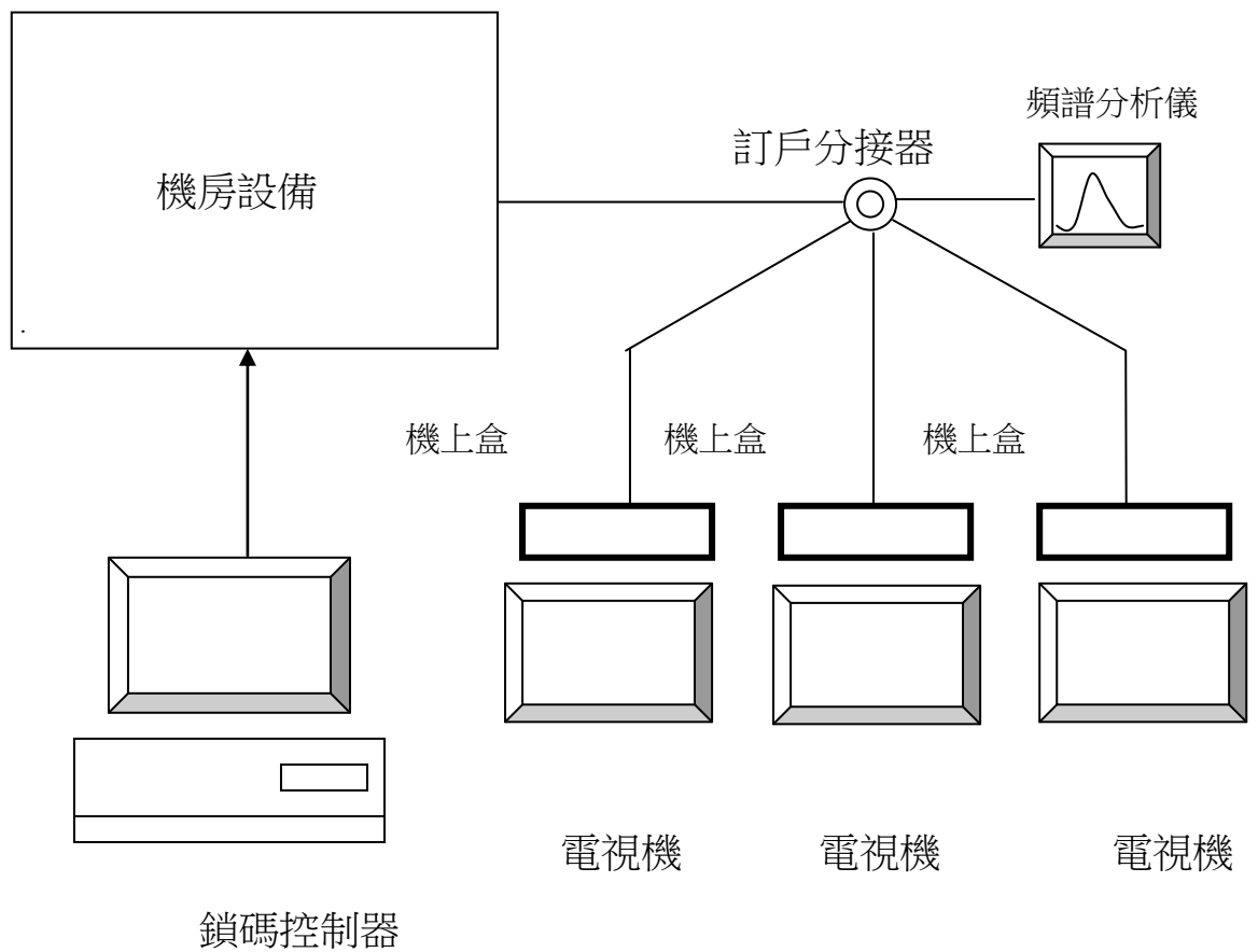
圖 11 定址鎖碼測試裝置
