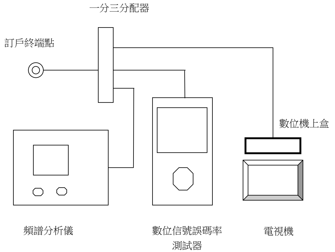
圖 12 測量數位有線電視誤碼率之測試裝置
