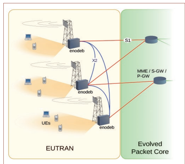
圖1 ▶ LTE網路架構（圖片來源：維基百科）
