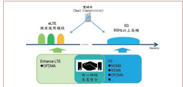
圖5 5G存取網路架構
