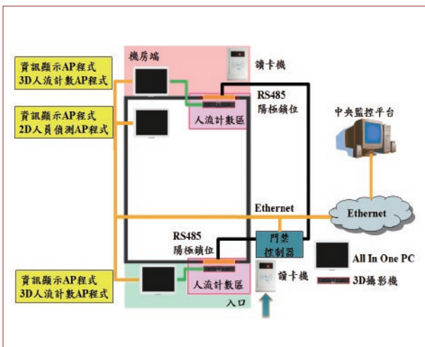
圖6 人流計數防尾隨架構
