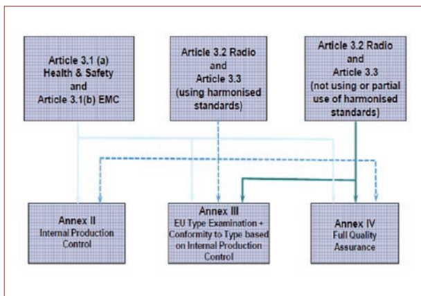
圖4 歐盟RED指令2014/53/EU CAB符合性評估流程
