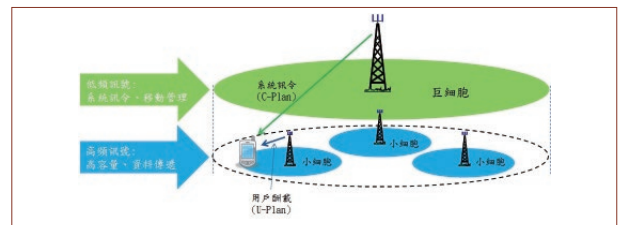
圖6 階層式細胞涵蓋
