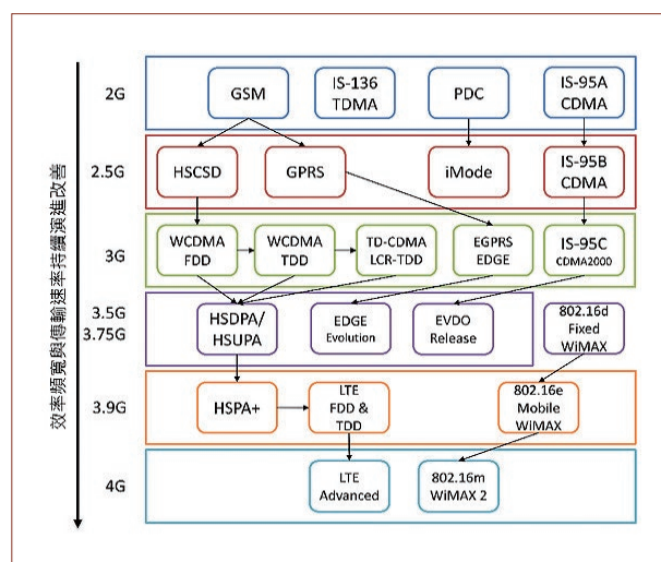
圖1 行動通訊標準演進
