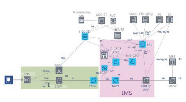
圖2 ● VoLTE網路架構（圖片來源：台灣大哥大）
