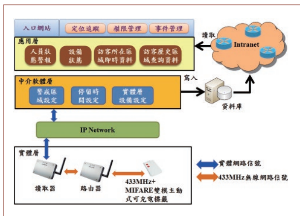
圖1 人員定位功能架構
