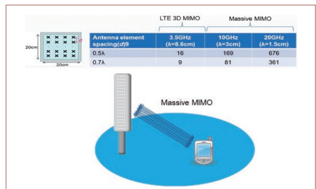
圖7 多天線陣列、多輸入輸出 (資料來源：NTT DOCOMO)
