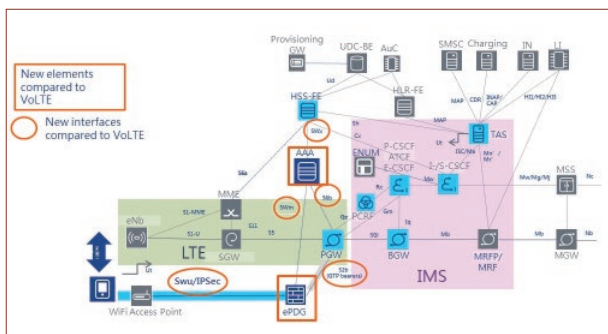
圖3 ● VoWiFi網路架構（圖片來源：台灣大哥大）
