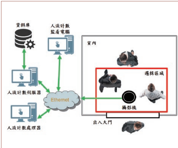
圖5 人流計數架構圖
